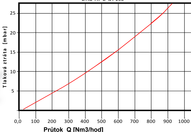
DRUCKVERLUSTTABELLE DER DETONATIONS - ROHR SICHERUNG DAG-A7-B-IIA-150
