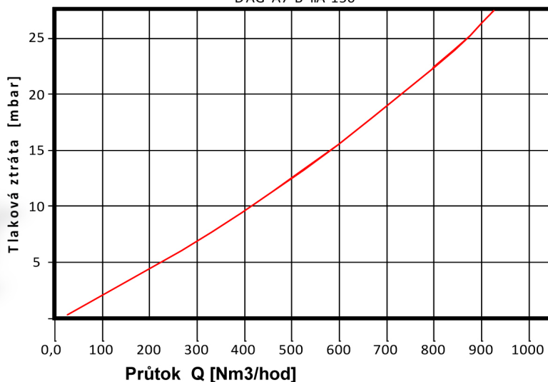
TLAKOVÁ ZTRÁTA PROTIEXPLOZNÍ POJISTKY DAG-A7-B-IIA-150
